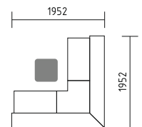
VR19H UKŁAD LADY/RECEPTION DESK SYSTEM 1952/1952/1100
